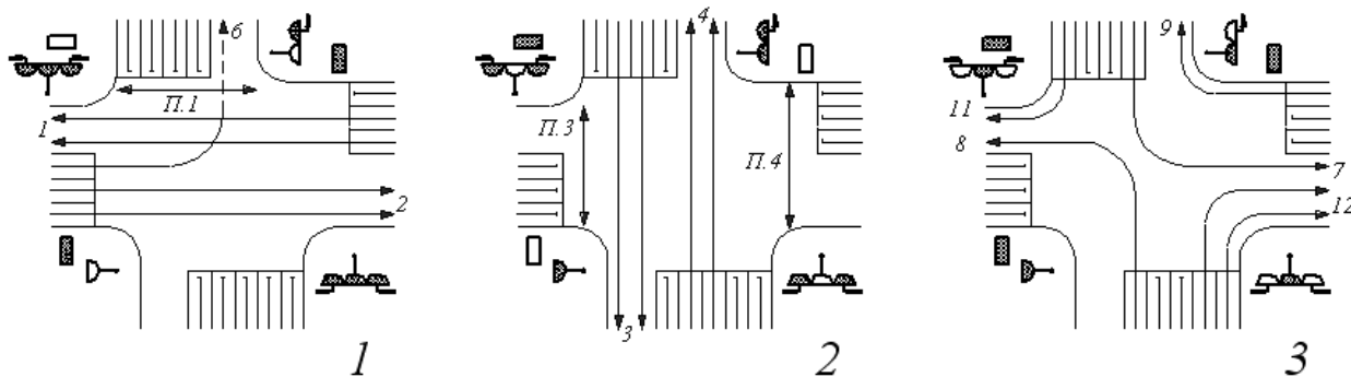
Рис. 1. Организация движения на перекрестке: пофазный принцип управления движением
